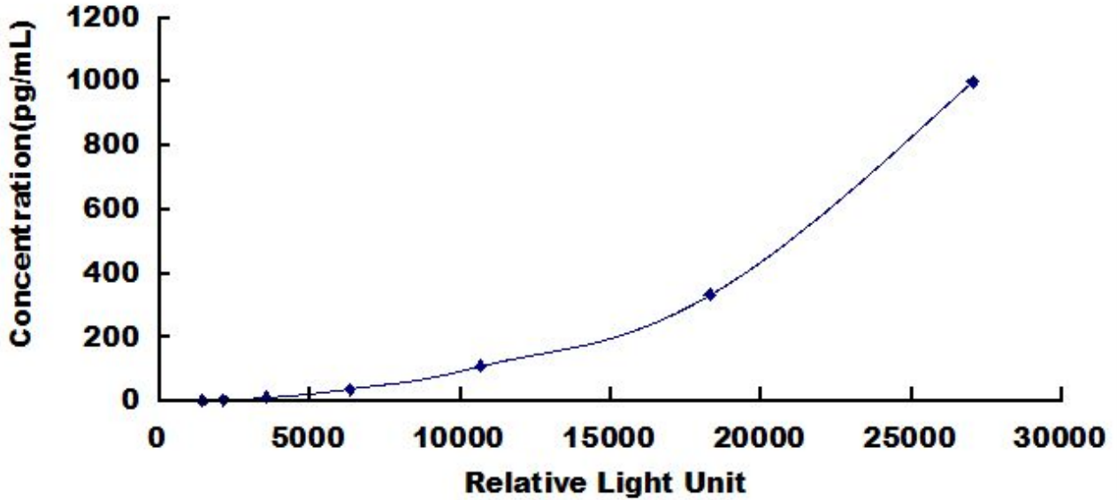
人抑制素 β E (INHbE) 检测试剂盒标准曲线
