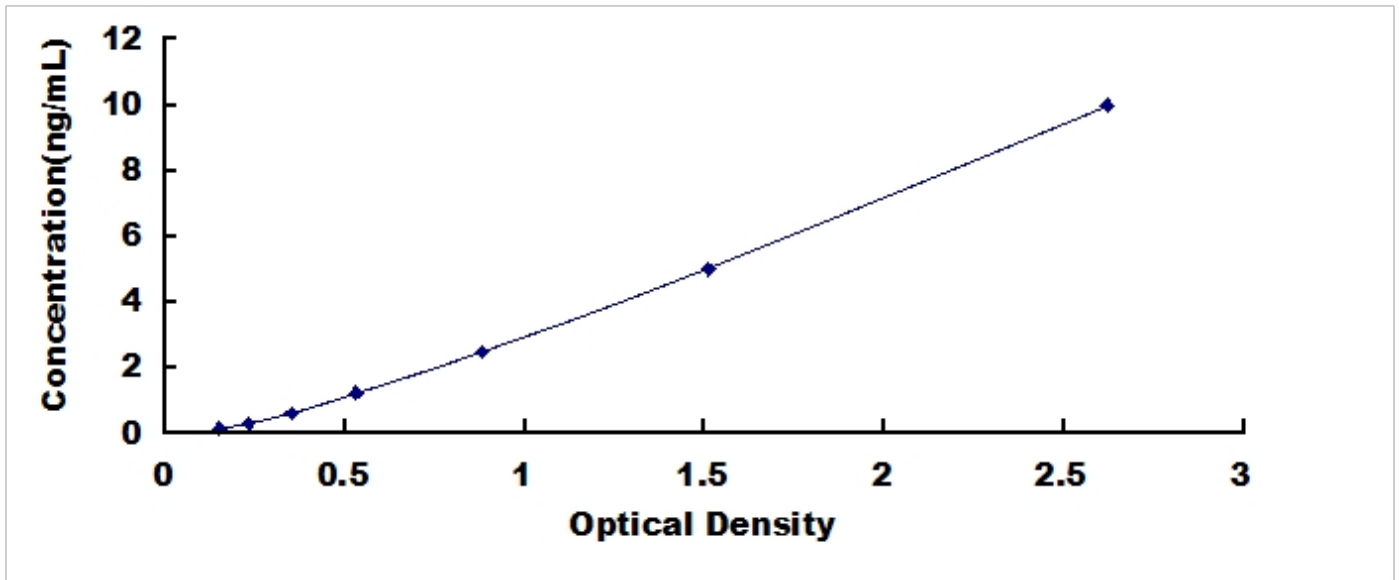
人 5-羟色胺受体 2A (HTR2A) 检测试剂盒标准曲线
