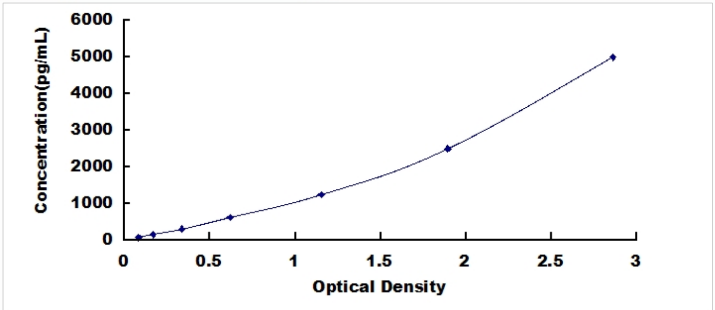
人酰基辅酶 A 合成酶长链家族成员 3 (ACSL3) 检测试剂盒标准曲线
