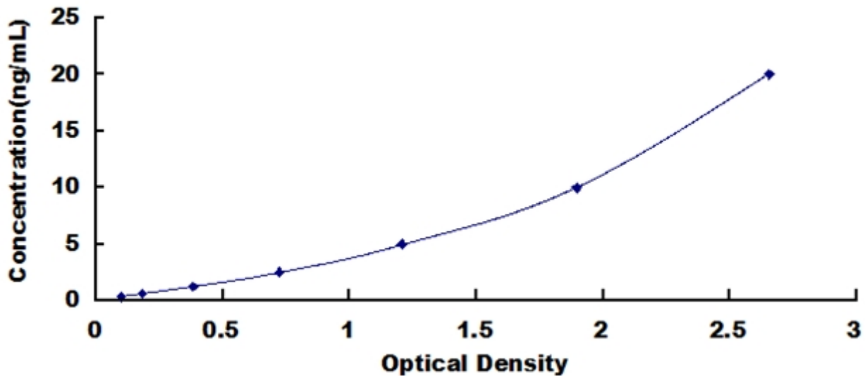
人二磷酸甘油酸变位酶 (BPGM) 检测试剂盒标准曲线
