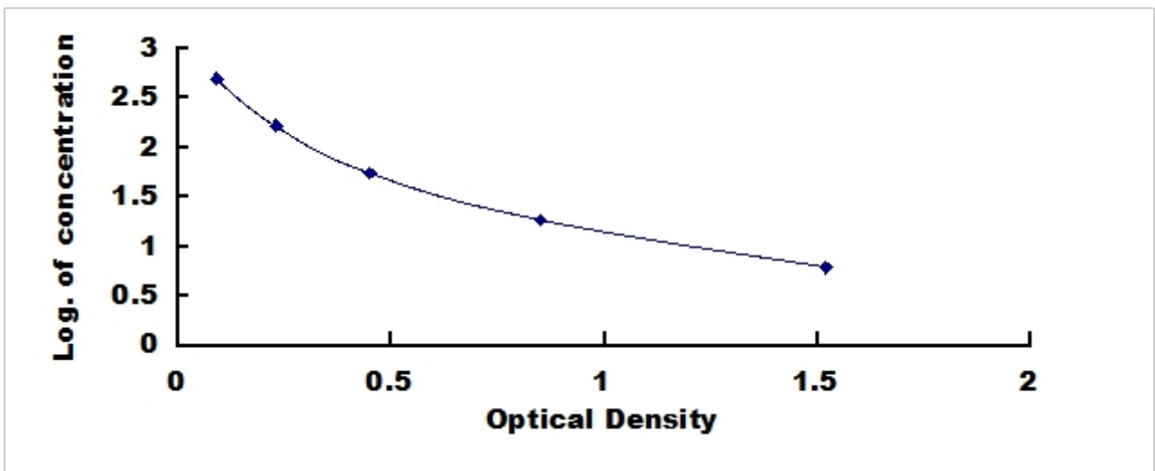
胆固醇(CH)检测试剂盒标准曲线
