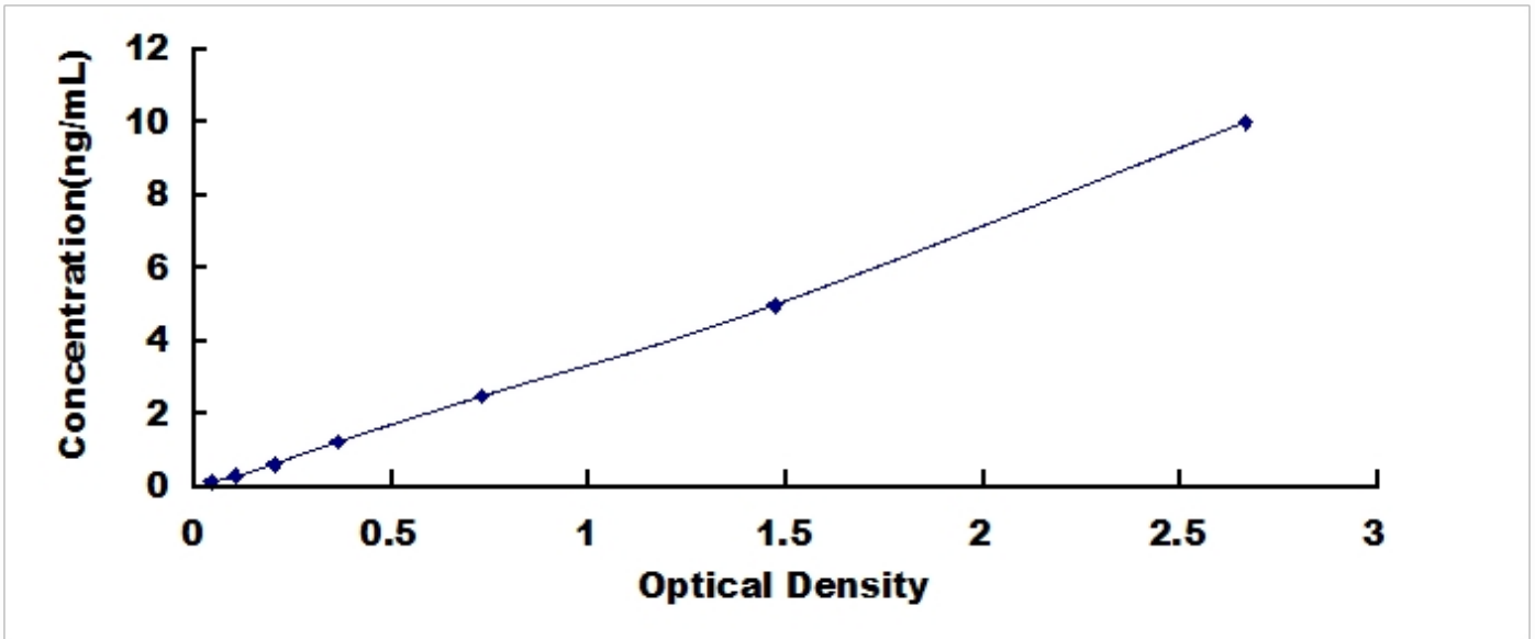
人 DNA 甲基转移酶 3 样蛋白 (DNMT3L) 检测试剂盒标准曲线
