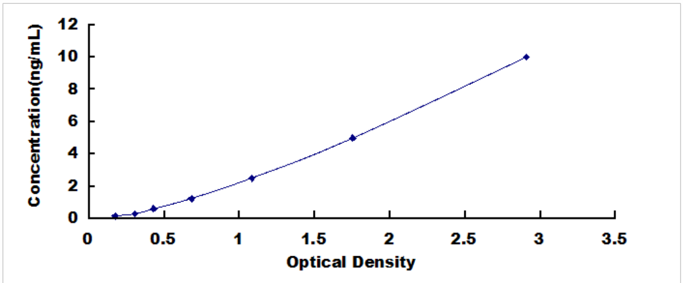
人成纤维细胞生长因子受体 3 (FGFR3) 检测试剂盒标准曲线
