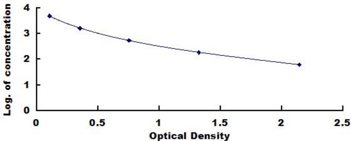
大鼠胃泌素抑制肽(GIP)检测试剂盒标准曲线
