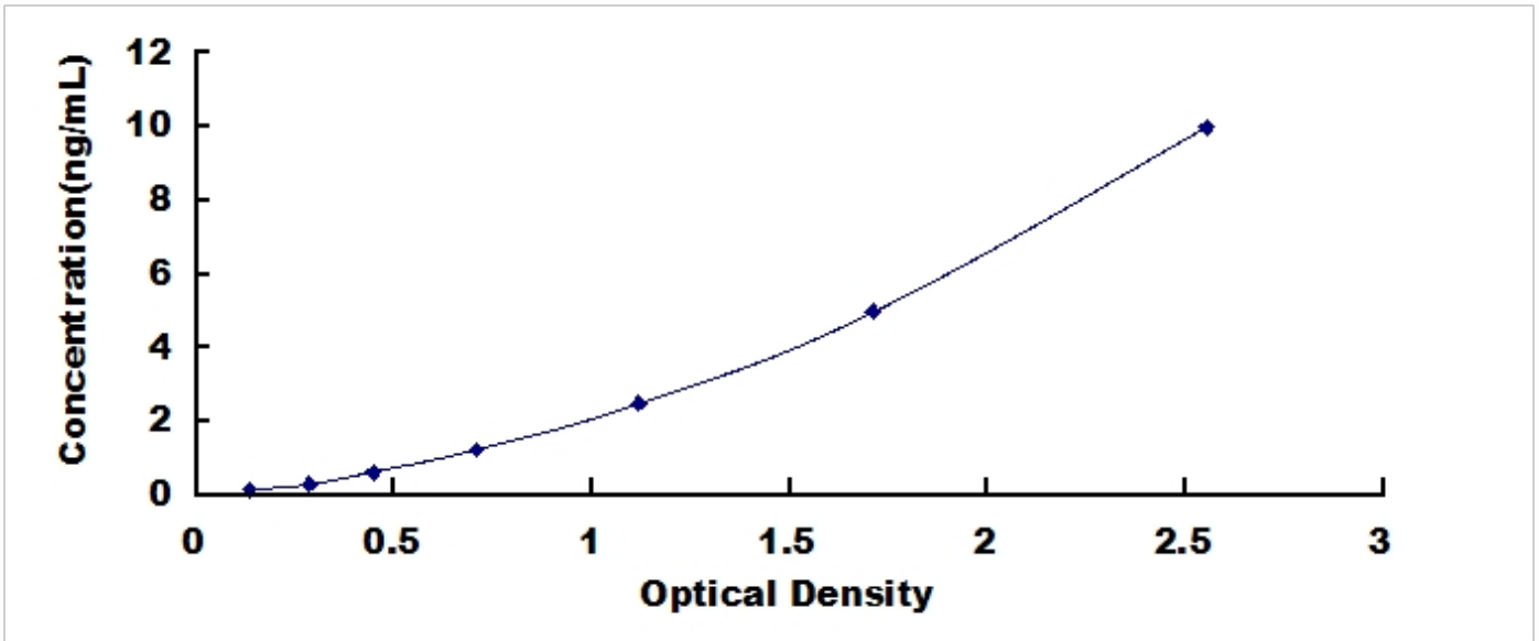
人热休克转录因子 1 (HSF1) 检测试剂盒标准曲线
