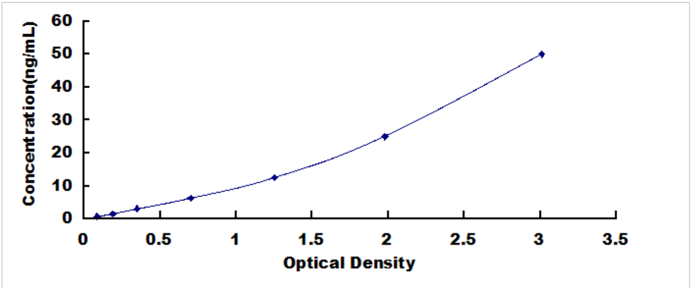
人氨基己糖苷酶 B \beta (HEXb) 检测试剂盒标准曲线
