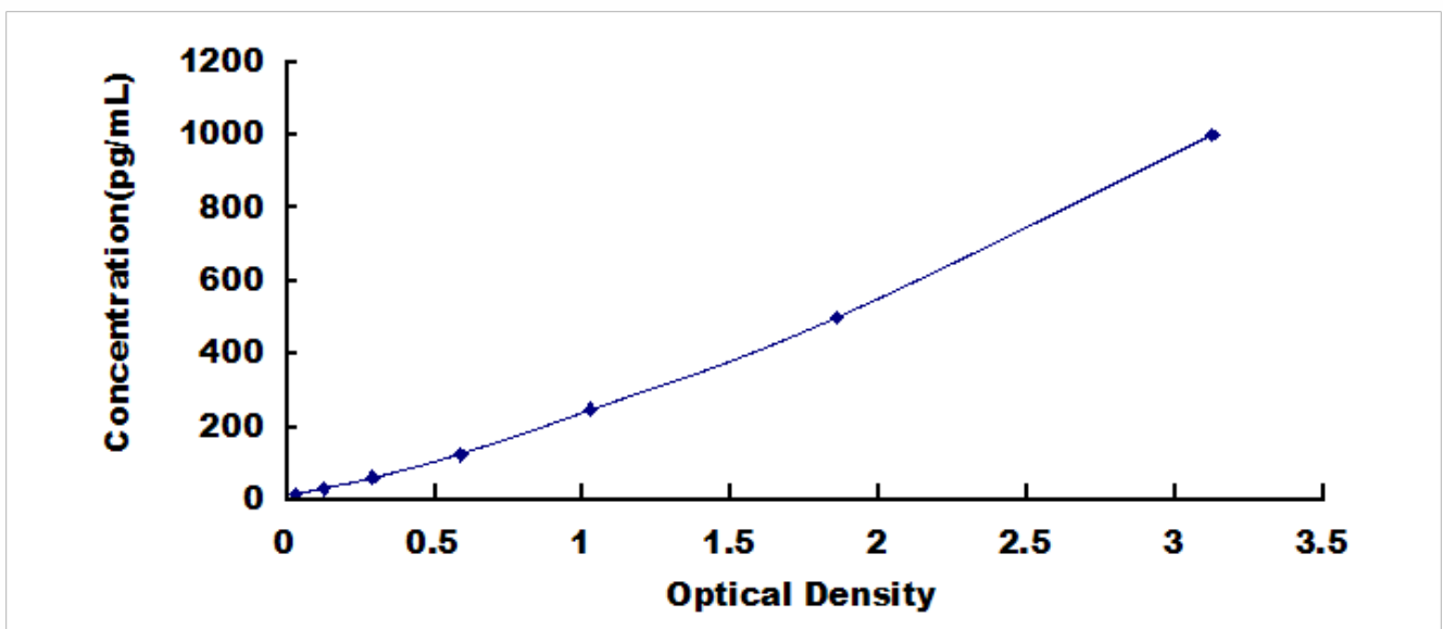
鸡胰岛素样生长因子结合蛋白 2(IGFBP2)检测试剂盒标准曲线
