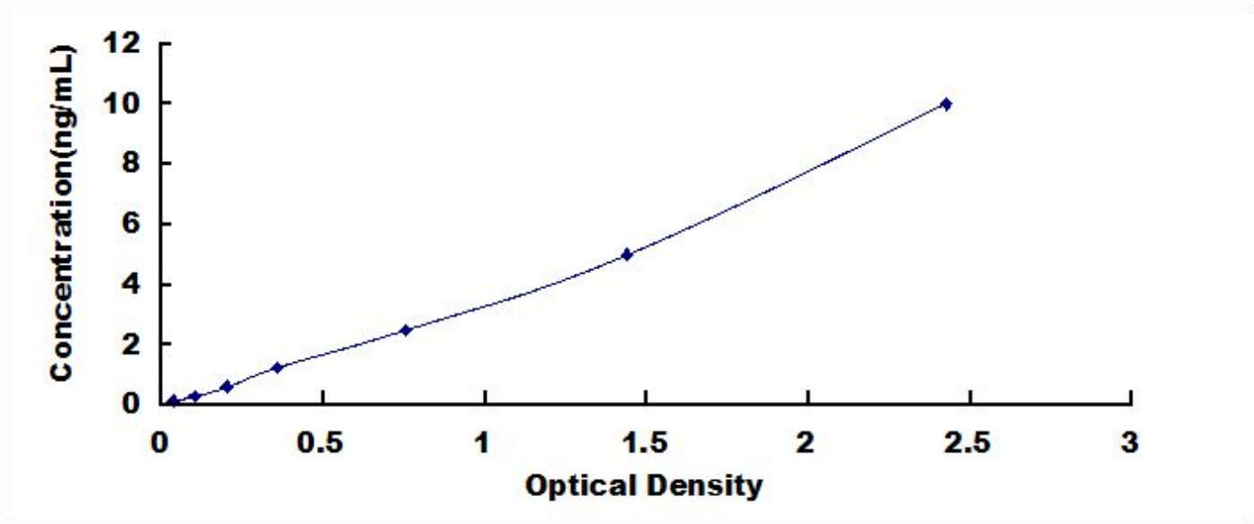
人染色质 SWI/SNF 相关基质关联肌动蛋白依赖性调节因子亚家族 C 成员 1 (SMARCC1) 检测试剂盒标准曲线
