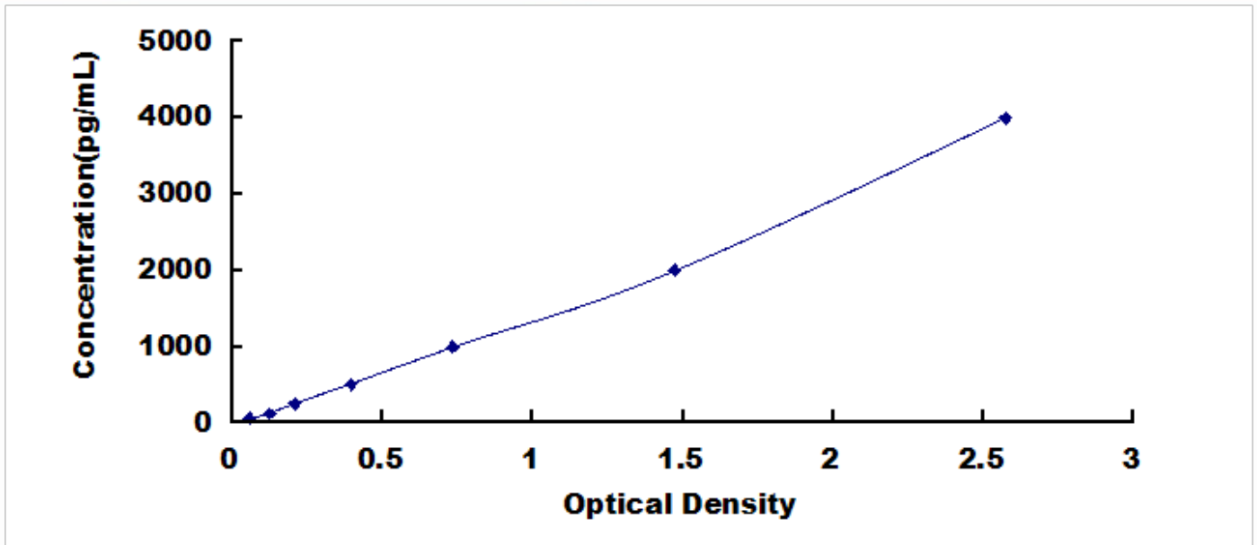
人分泌性白细胞蛋白酶抑制因子(SLPI)检测试剂盒标准曲线
