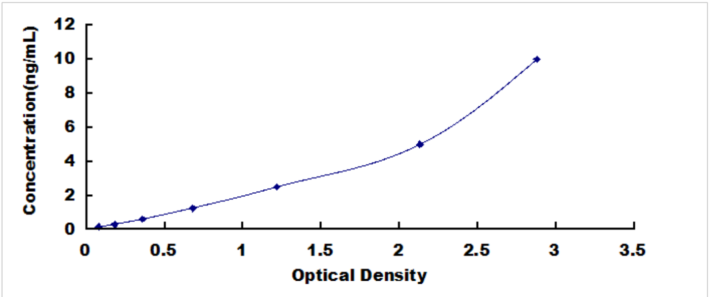
人分拣连接蛋白 17 (SNX17) 检测试剂盒标准曲线
