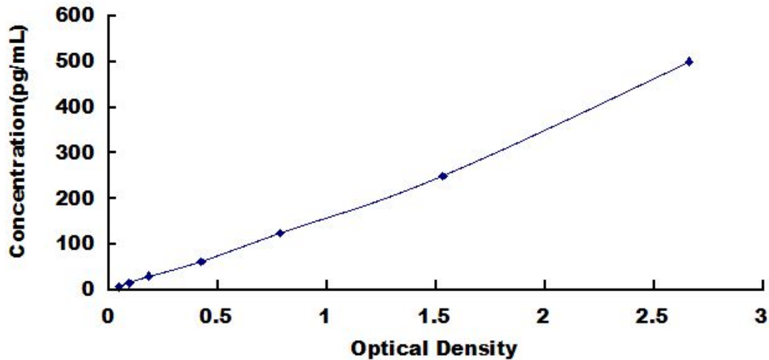
小鼠类胰蛋白酶(TPS)检测试剂盒标准曲线
