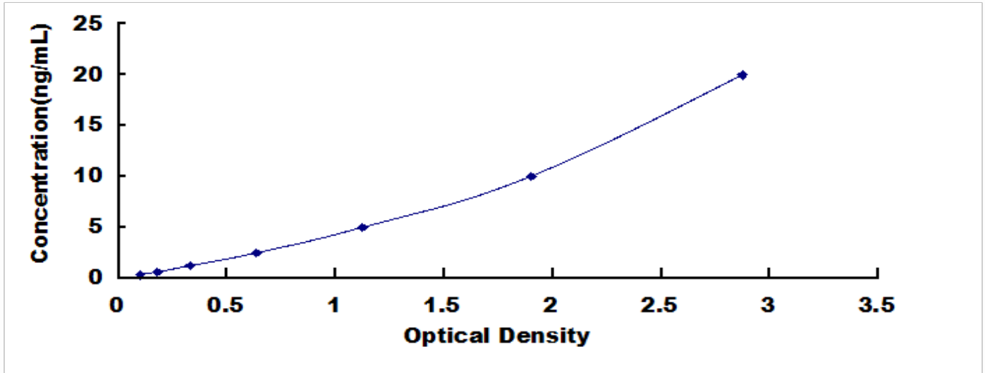
人结合珠蛋白 (Hpt) 检测试剂盒标准曲线
