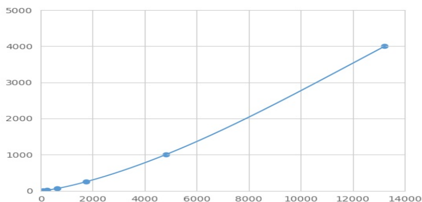
(甲胎蛋白)检测试剂盒标准曲线
