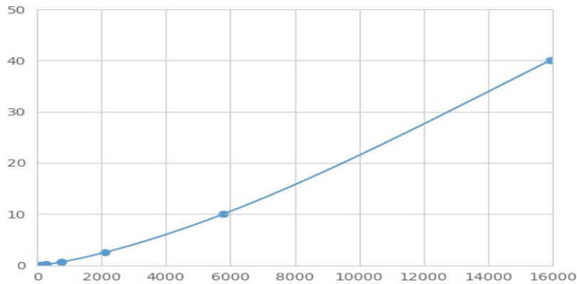
(血管生成素样蛋白6)检测试剂盒标准曲线
