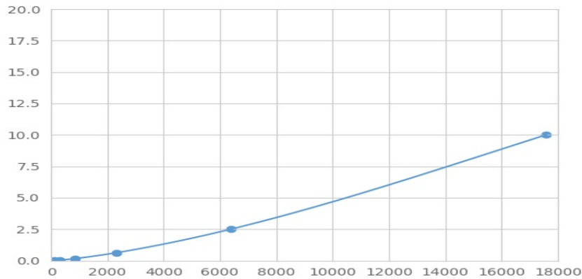
(天冬氨酸β羟化酶)检测试剂盒标准曲线
