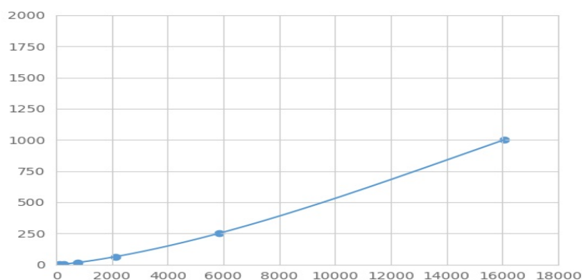
(和肽素) 检测试剂盒标准曲线
