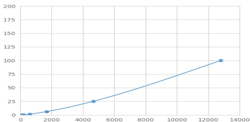
(纤维蛋白原 \alpha )检测试剂盒标准曲线
