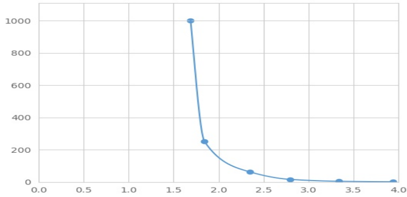
(胰高血糖素样肽1)检测试剂盒标准曲线
