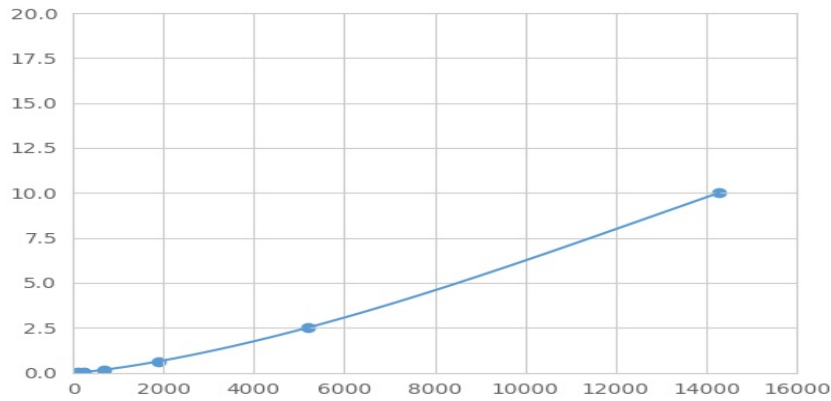
(糖原磷酸化酶L) 检测试剂盒标准曲线
