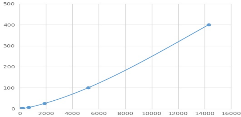
(激肽释放酶结合蛋白)检测试剂盒标准曲线
