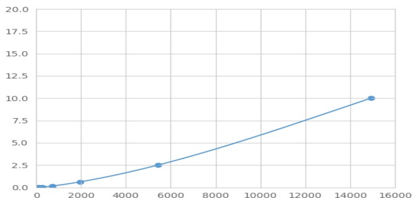
(N-乙酰转移酶1) 检测试剂盒标准曲线
