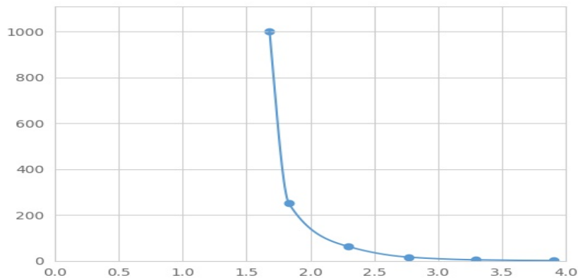
(神经介素B)检测试剂盒标准曲线
