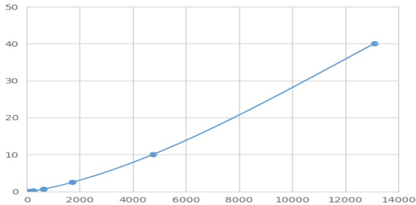
(前胶原C端蛋白酶增强子)检测试剂盒标准曲线
