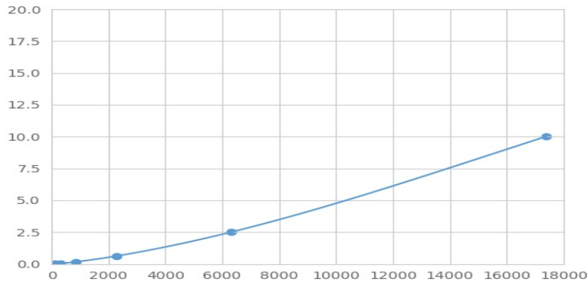
(原卟啉原氧化酶)检测试剂盒标准曲线
