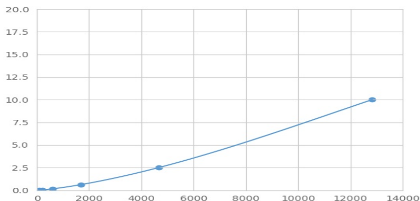
(维甲酸受体 \gamma ) 检测试剂盒标准曲线
