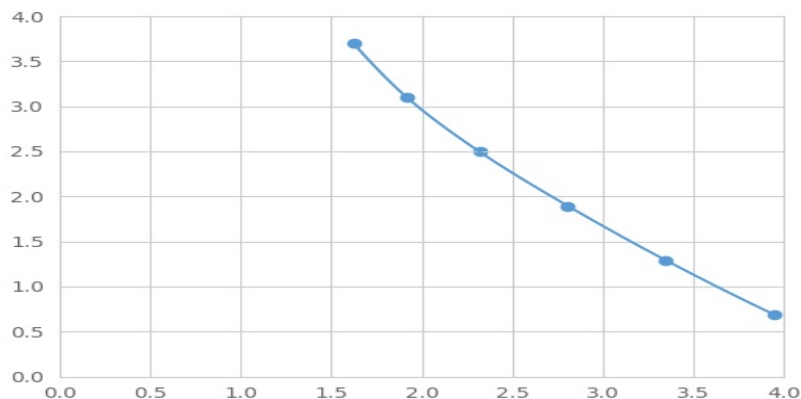
(促泌素)检测试剂盒标准曲线
