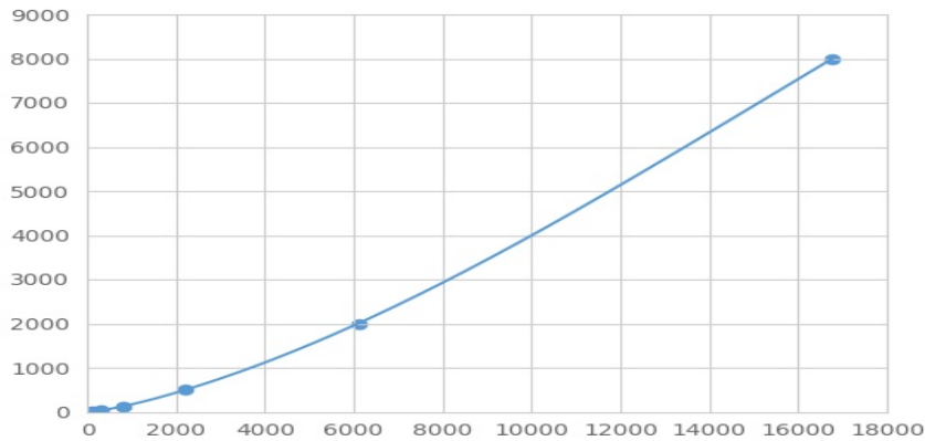
(胞外超氧化物歧化酶)检测试剂盒标准曲线
