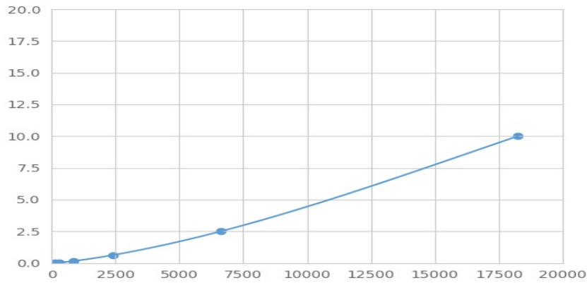
(原肌球蛋白3)检测试剂盒标准曲线
