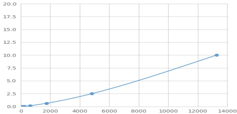
(肿瘤坏死因子受体超家族成员7)检测试剂盒标准曲线
