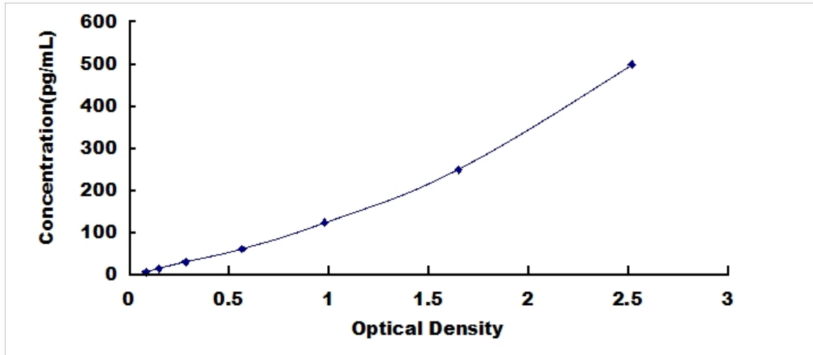
人巨噬细胞集落刺激因子(MCSF)检测试剂盒标准曲线
